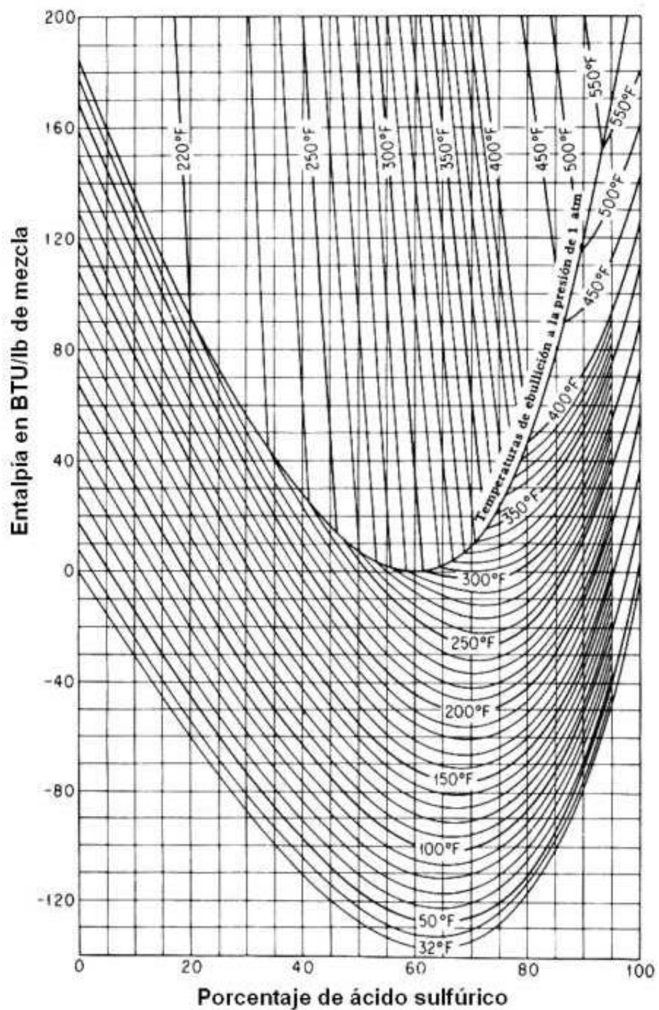
Diagrama entalpia - composición para el sistema ácido sulfúrico - agua. Estados de referencia: agua líquida y ácido sulfúrico a 32° F y a sus presiones de vapor correspondientes
