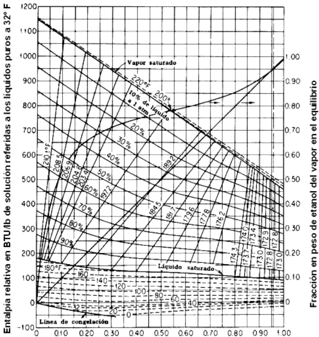
Fracción en peso de etanol en las mezclas de etanol - agua Diagrama de entalpia - concentración para el sistema etanol - agua, mostrando las fases de líquido y vapor a 1 atm. de presión total.
