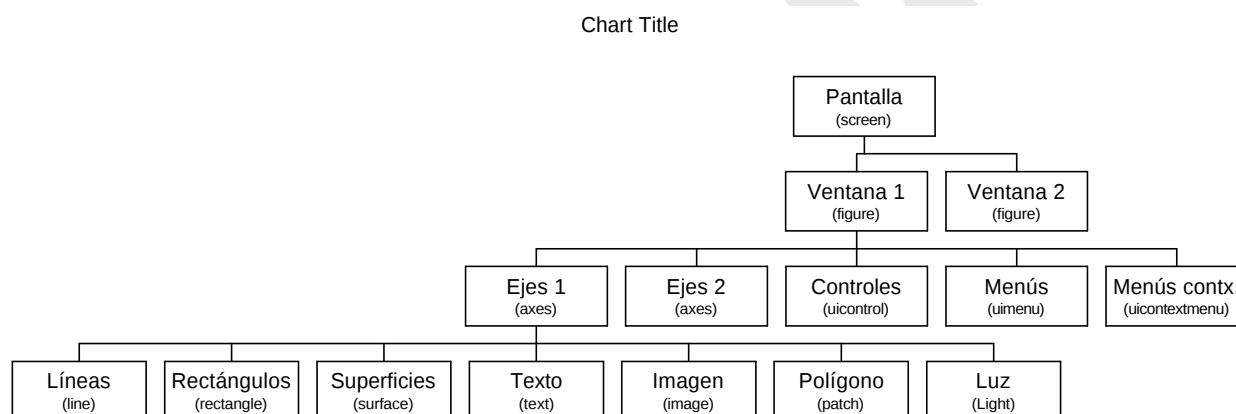
Figura 24. Jerarquía gráfica de MATLAB.
