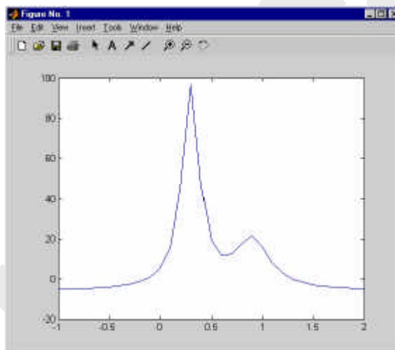
Figura 22. Función "prueba".
