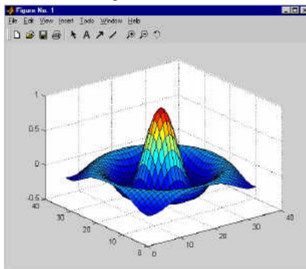
Figura 19. Función “sombrero” con facetas.
