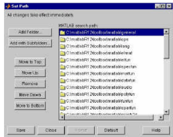
Figura 6. Path Browser .
