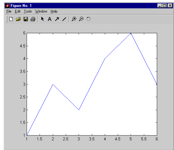
Figura 14. Gráfico del vector x=[1\ 3\ 2\ 4\ 5\ 3] .
